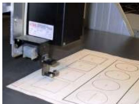
Hình 6.4: Máy vẽ
