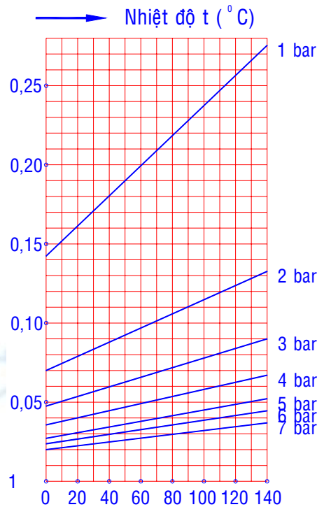
Hình 1. Sự phụ thuộc áp suất, nhiệt độ và độ nhớt động của không khí.
